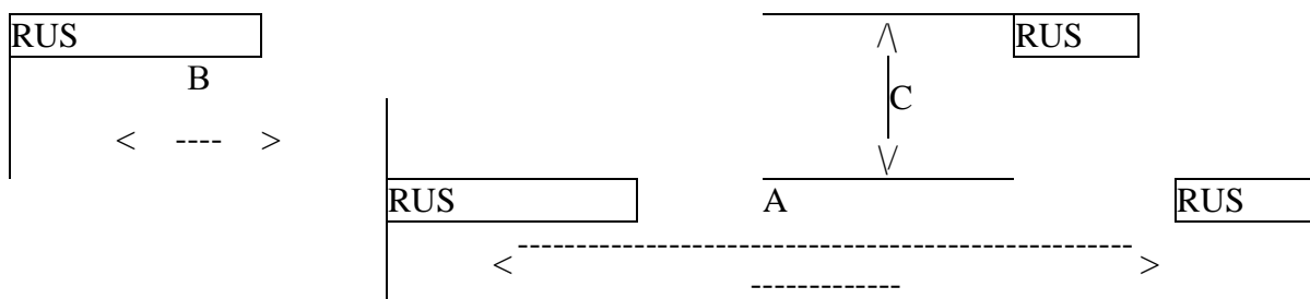
Рис. 1. Фрагмент размещения защитных элементов (А - интервал между элементами в горизонтальном ряду; В - смещение рядов защитных элементов по горизонтали относительно друг друга; С - расстояние между рядами)
